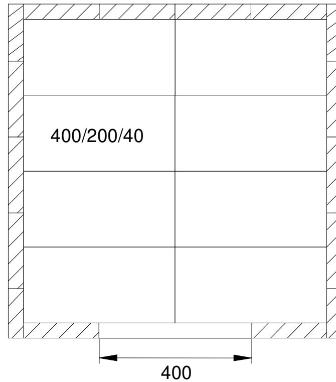
Bodenansicht (Querschnitt)
